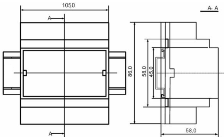
Рисунок 3 – Габаритные и присоединительные размеры блока питания PSM-72-24
